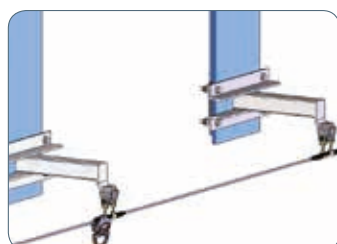
Fixation par bridage sur structure métallique
